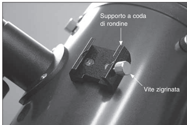
Figura 2: particolare della base del cercatore
