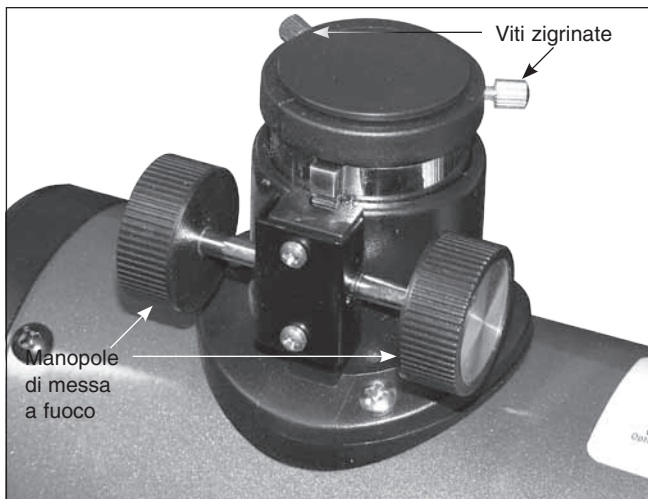
Figura 8: particolare del focheggiatore del telescopio da tavolo da 100 mm
