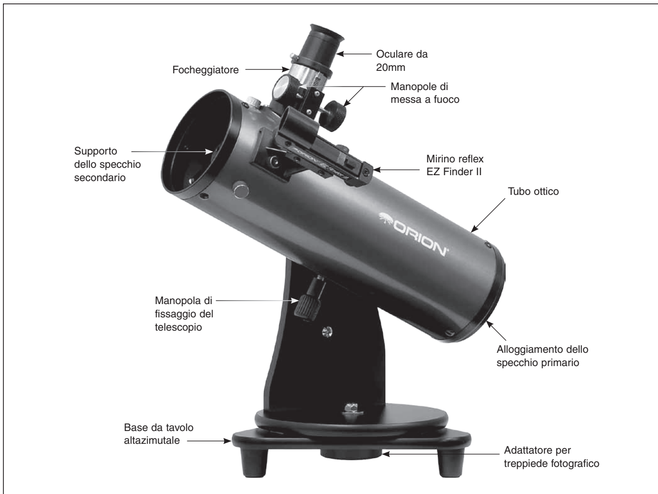
Figura 1a: telescopio da tavolo SkyScanner 100
