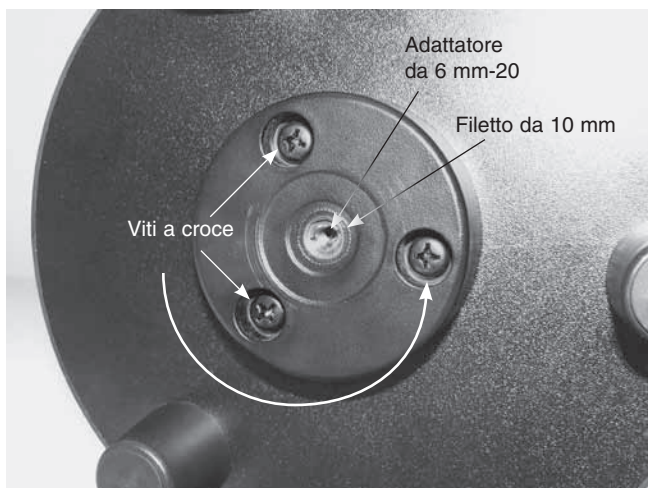
Figura 9a: particolare dell'adattatore per treppiede fotografico
