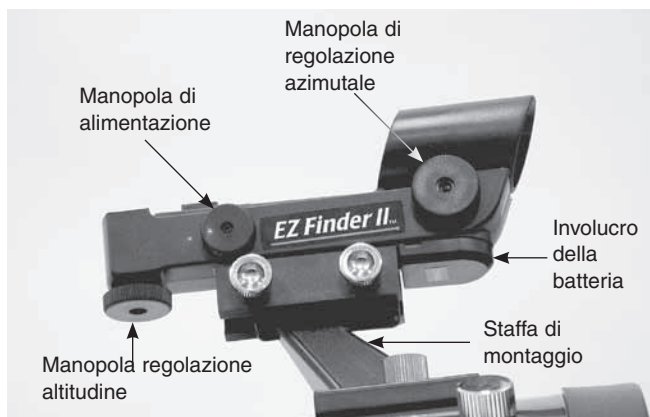
Figura 4: mirino reflex EZ Finder II.
