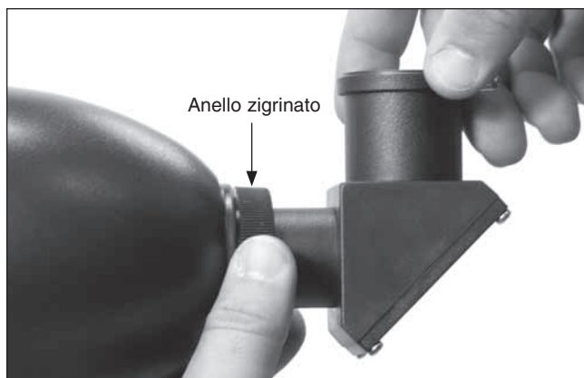
Figura 6: l'anello zigrinato del diagonale si collega ai filetti nella parte posteriore del telescopio GoScope. Per cambiare l'angolo di visuale, allentare l'anello zigrinato, ruotare il diagonale, quindi serrare nuovamente l'anello.
