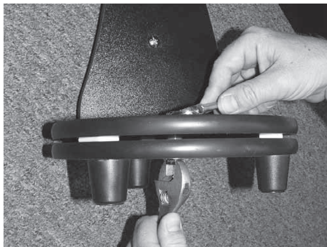
Figura 11: regolazioni opzionali alla tensione azimutale
