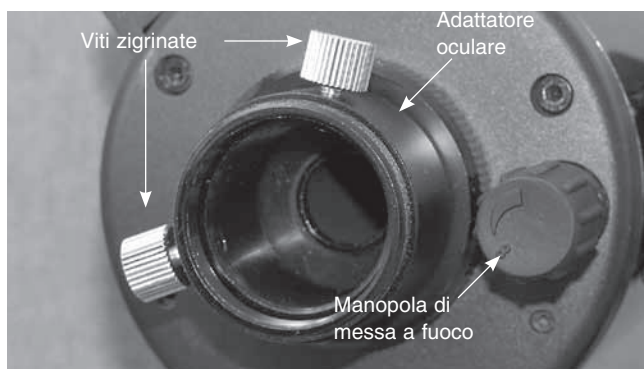
Figura 7: particolare dell'adattatore oculare del telescopio da tavolo da 90 mm
